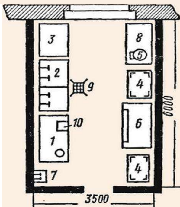
Схема 2. Примерная расстановка оборудования в рыбном. цехе:
